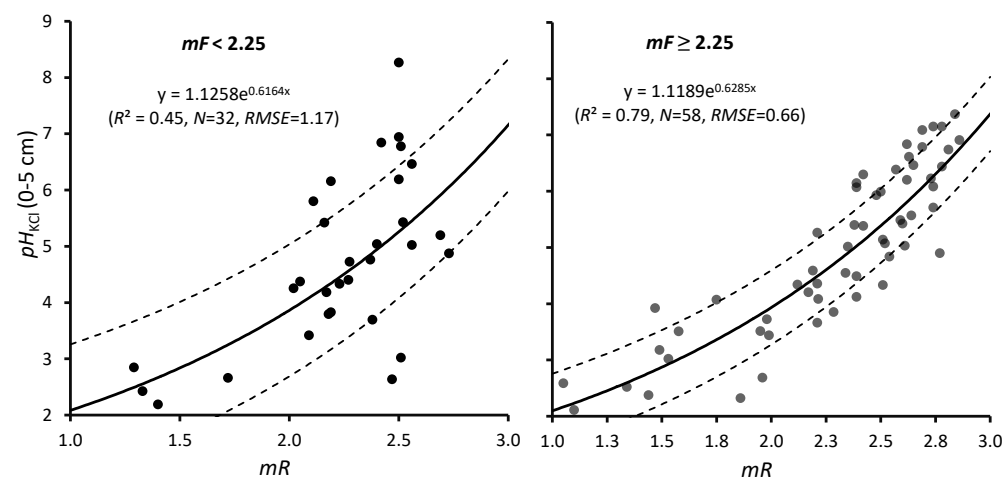
Figuur 5. Relatie tussen opnamegemiddelde zuurindicatie R_m en de \text{pH}_{\text{KCl}} in de bovenste bodemlaag (0-5 cm) van natte bodems (links) en van vochtige tot droge bodems (rechts). Bron: Witte et al. (2014), gegevens Cirkel et al. (2014b).
